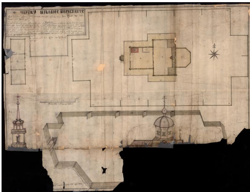
Рисунок 1. Чертеж Петропавловской церкви 1750 год
